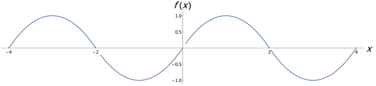
Figure 2: Função f(x) = 1 - (x - 1)^2 se 0 < x < 1 , 4-periódica, ímpar e simétrica com respeito ao eixo x = 1
