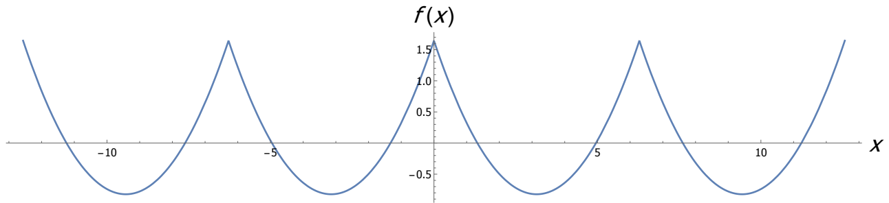
Figure 1: Função f(x) = \frac{1}{4}(x - \pi)^2 - \frac{\pi^2}{12} se 0 < x < \pi , 2\pi -periódica e par
