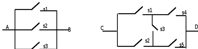
Figura 1: Problema 4: Circuitos em sistema de comunicação
